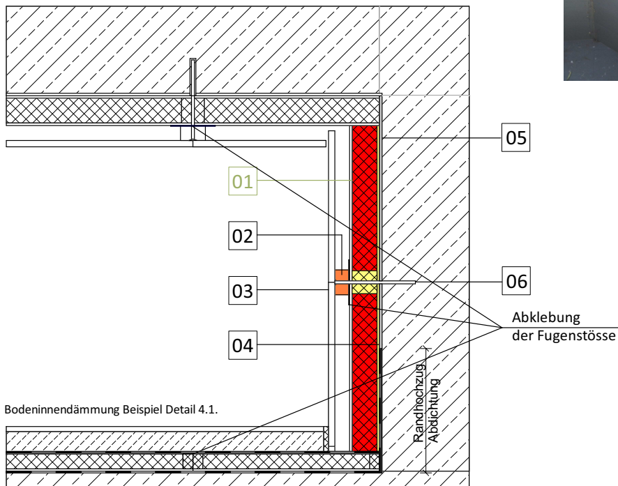
Deckeninnendämmung: Beispiel Detail 4.8.
